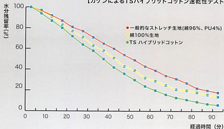
【カケンによるTSハイブリッドコットン速乾性テスト】
